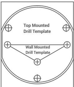
Bohrschablone (×1)
